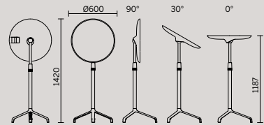
Tavolino regolabile in altezza con top rotondo ø 600 mm
