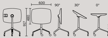
Tavolino regolabile in altezza con top rotondo ø 600 mm
