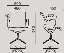
Meeting su base 5 razze e braccioli
