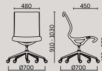
Meeting su base 4 razze e braccioli
