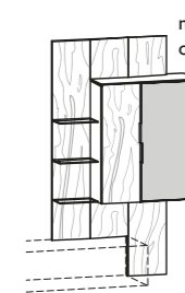
B/T/H 111,8/37,3/193,8 cm
